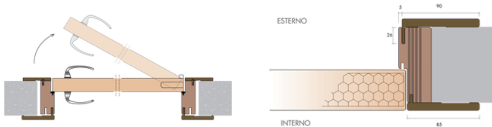
COMPLANARI CERNIERA A SCOMPARSA - FILO INTERNO
