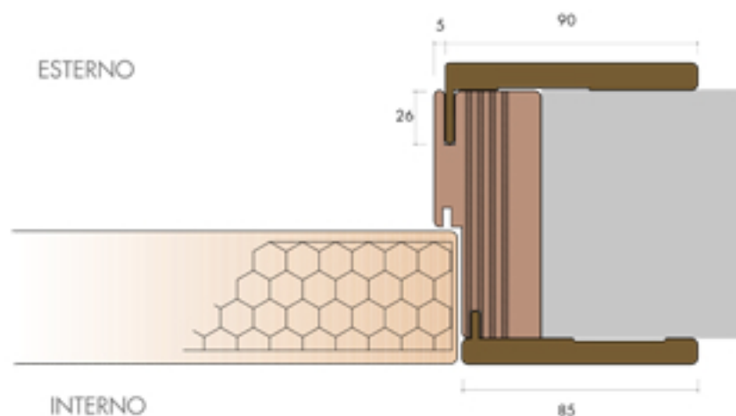
BATTENTE CERNIERA A SCOMPARSA - Filo Interno
