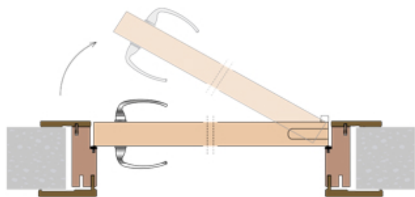
BATTENTE CERNIERA A SCOMPARSA - Filo Interno
