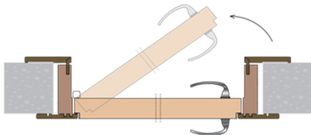
COMPLANARI CERNIERA A SCOMPARSA - FILO INTERNO
