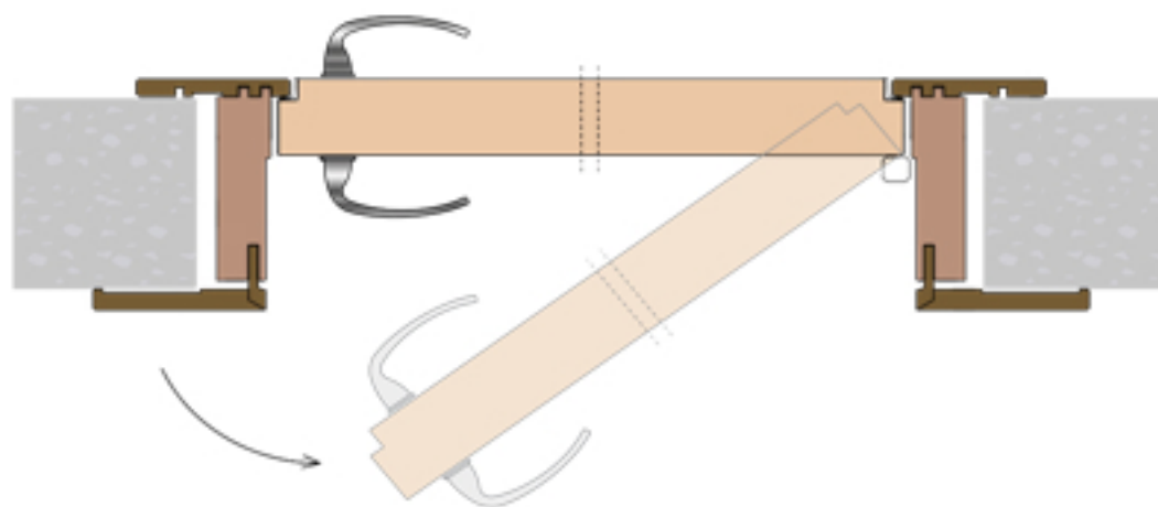
BATTENTE CERNIERA A SCOMPARSA - Filo Interno
